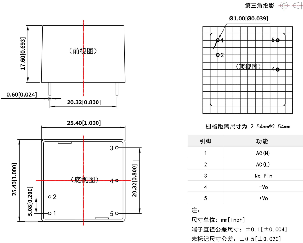
AD03-23Sxx-T 接线式封装外观尺寸
