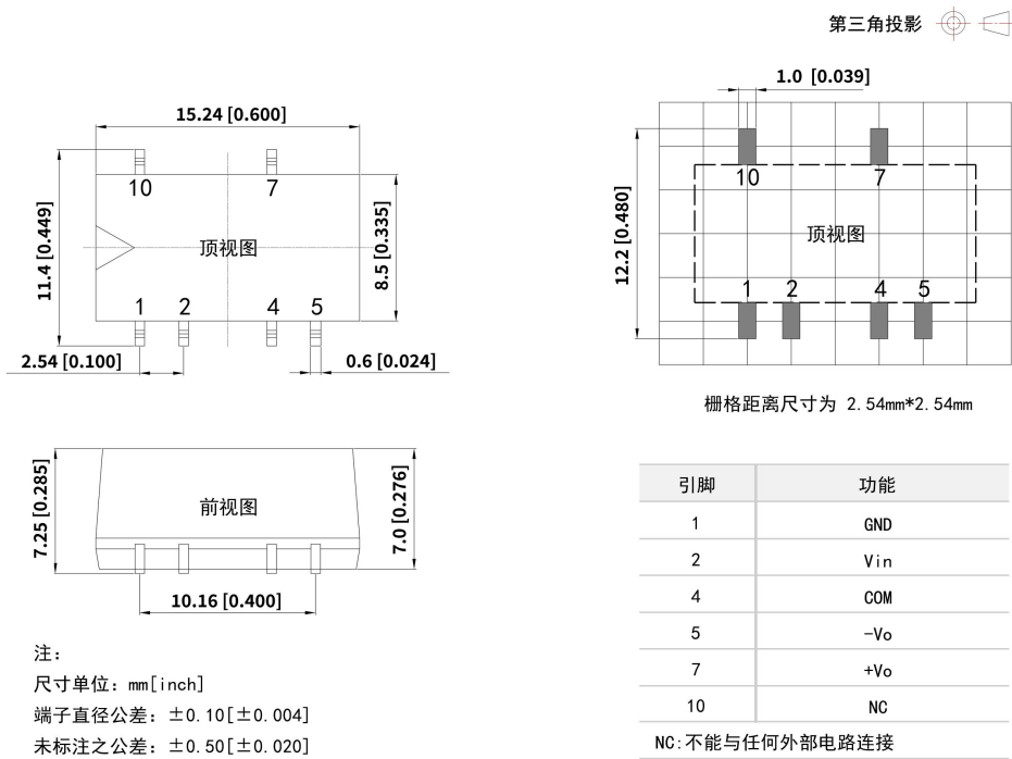
DB1-xxDxxXT 外观尺寸与建议刷版图
