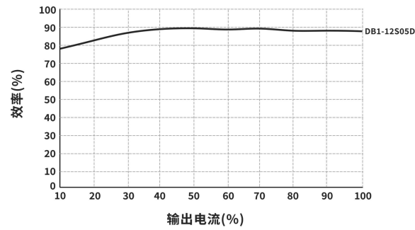
效率 VS 输出负载曲线图 (Vin=12V)
