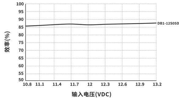
效率 VS 输入电压曲线图 (满载、Vin=12V)
