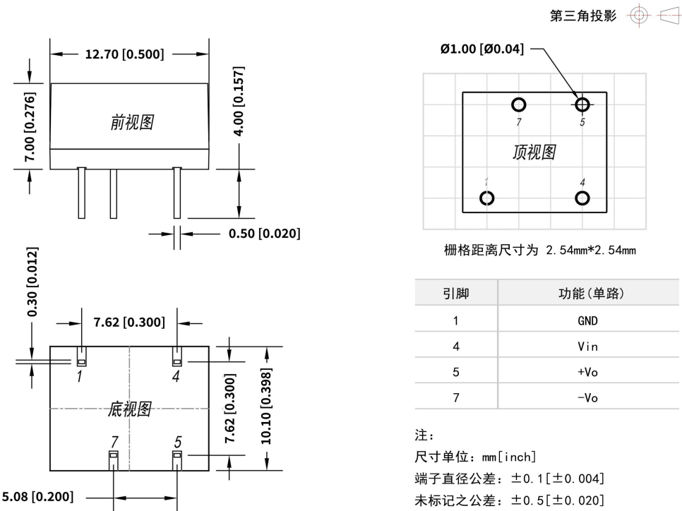
DB1-xxSxxD 外观尺寸与建议刷版图
