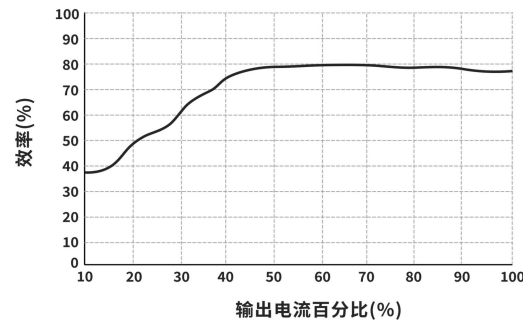
效率 VS 输出负载曲线图 (DB1-05S05S)
