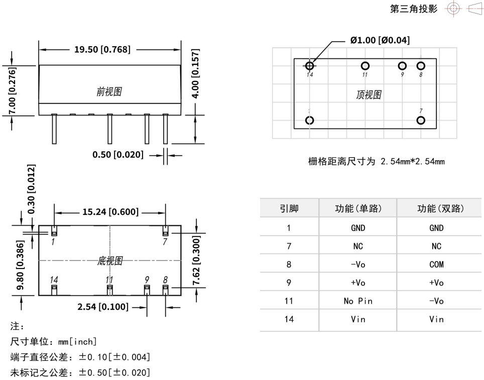
DB2-xxDxxD 外观尺寸与建议刷版图
