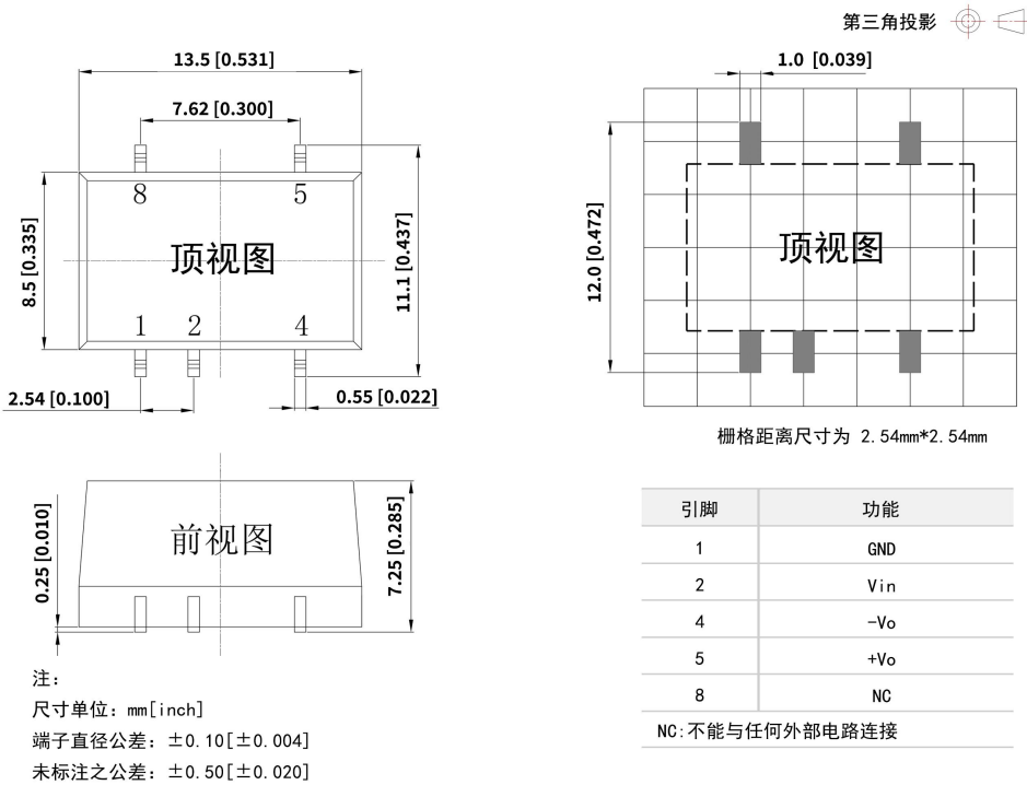
DB2-xxSxxXT 外观尺寸与建议刷版图
