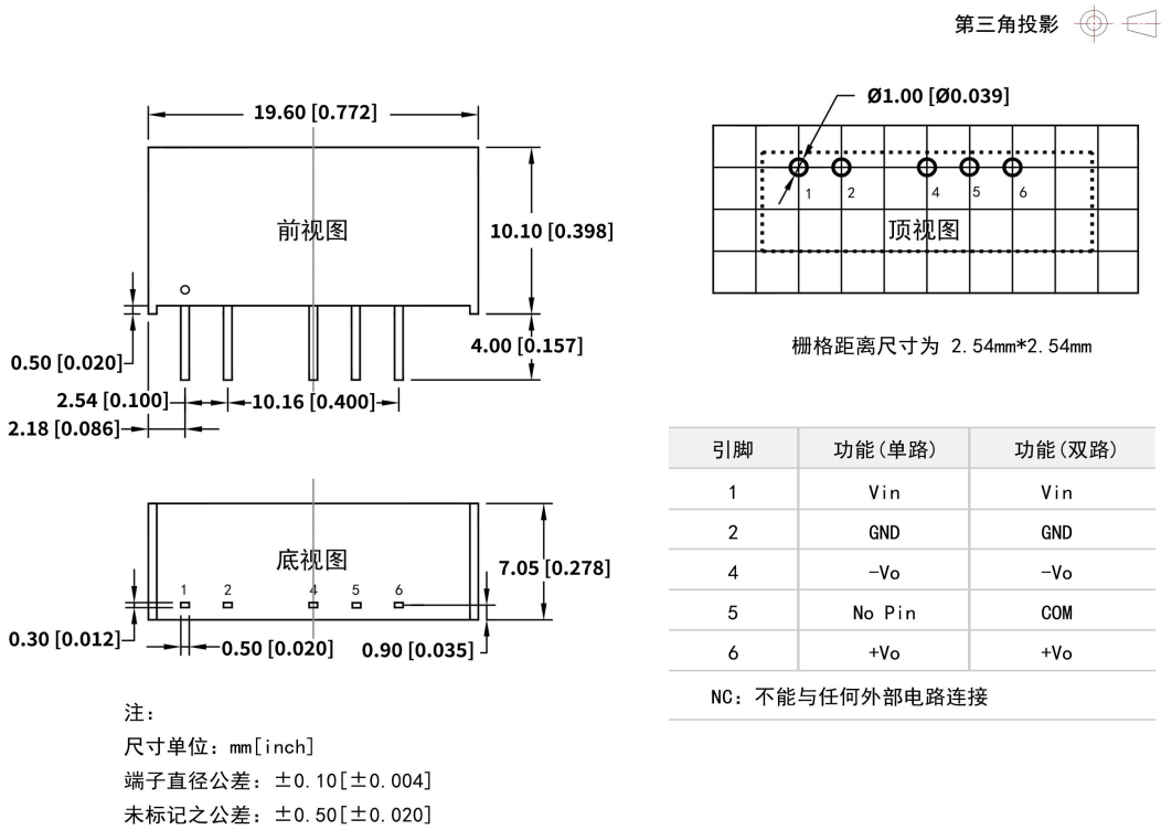
DB3-xxDxxLS 外观尺寸与建议刷版图
