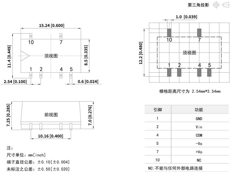
DF1-xxDxxXT 外观尺寸与建议刷版图
