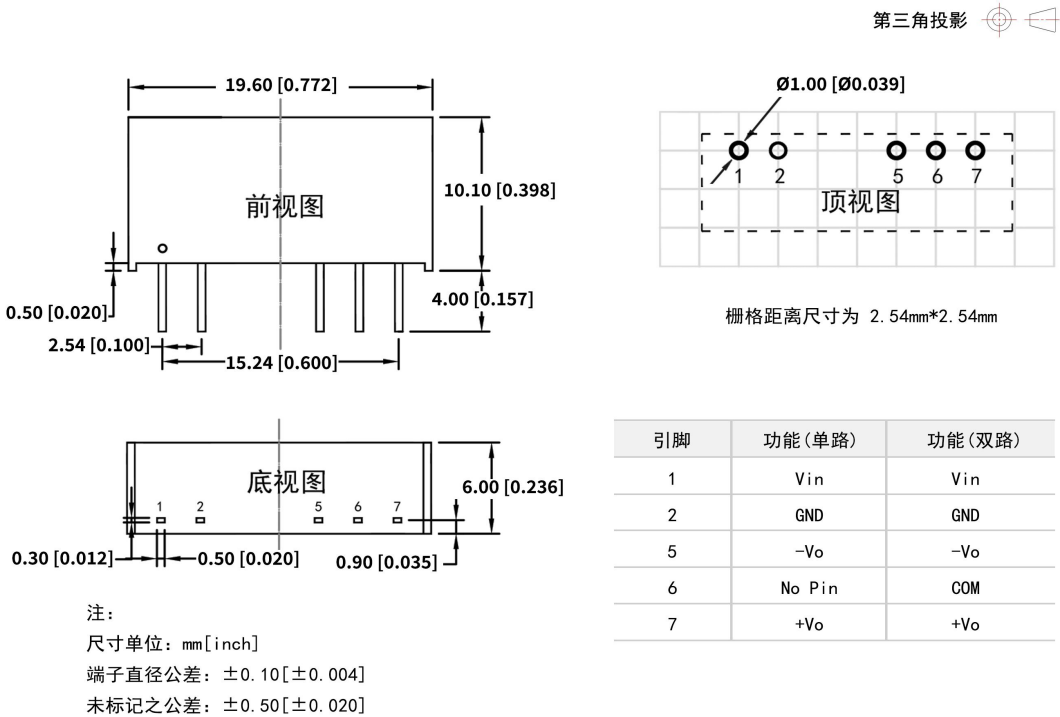
DF1-xxSxxLS 外观尺寸与建议刷版图
