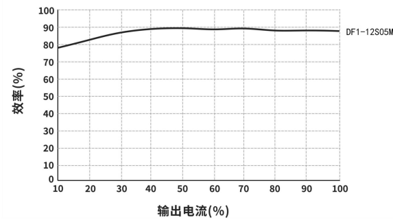
效率 VS 输出负载曲线图 (Vin=12V)
