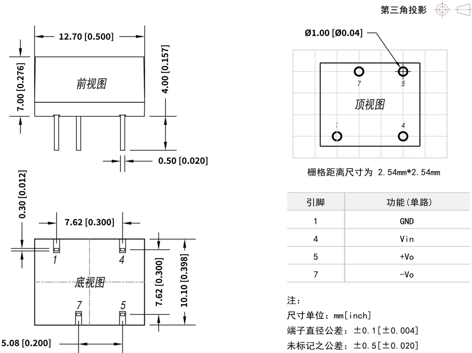
DF1-xxSxxM 外观尺寸与建议刷版图
