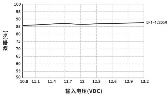
效率 VS 输入电压曲线图 (满载、Vin=12V)
