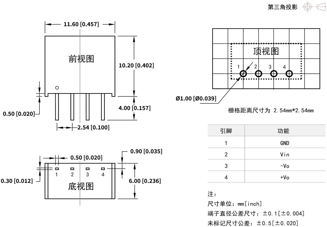
DF1-xxSxxS 外观尺寸与建议刷版图
