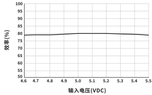
效率 VS 输入电压曲线图 (满载、DF1-05S05S)
