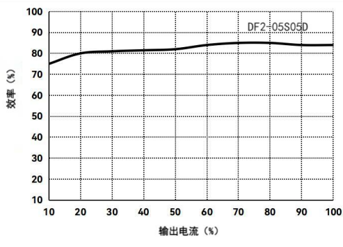
效率 VS 输出负载曲线图 (Vin=5V)
