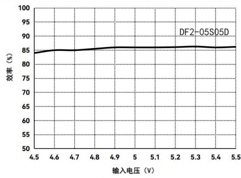
效率 VS 输入电压曲线图 (满载、Vin=5V)
