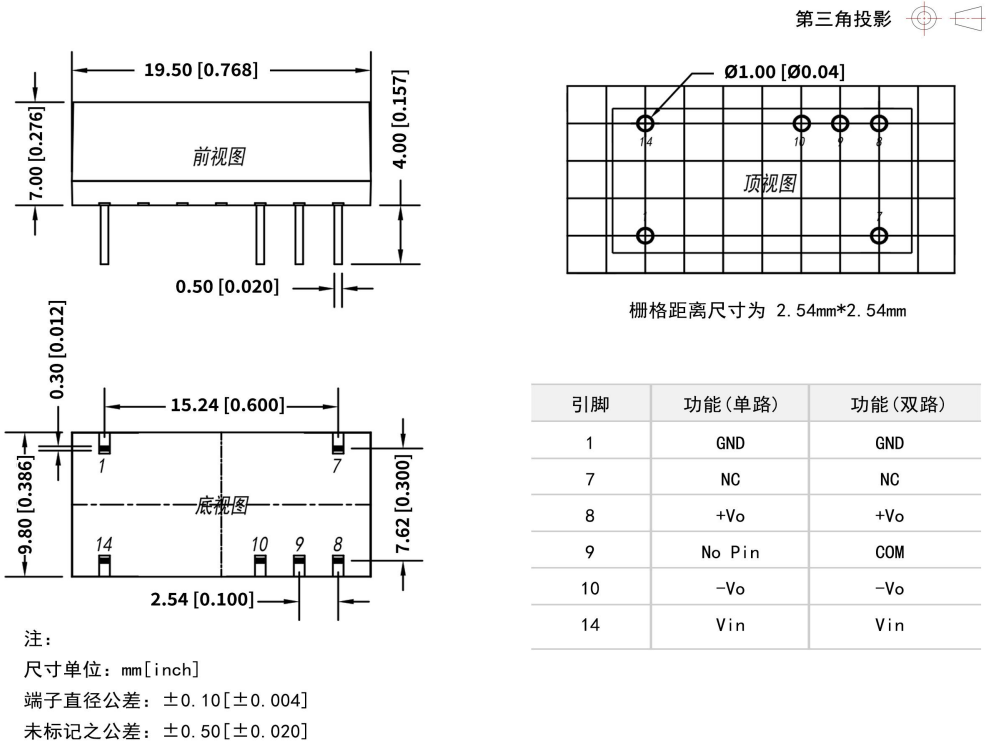
DF2-xxSxxD 外观尺寸与建议刷版图
