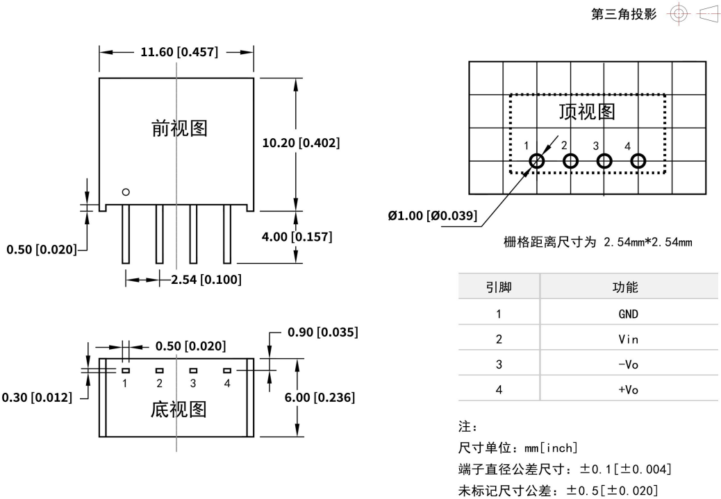
DF2-xxSxxS 外观尺寸与建议刷版图
