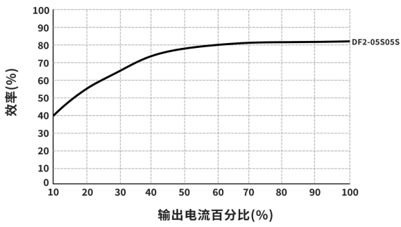
效率 VS 输出负载曲线图 (DF2-05S05S)
