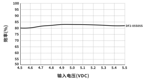
效率 VS 输入电压曲线图 (满载、DF2-05S05S)
