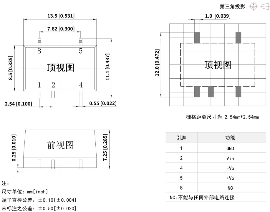
DF2-xxSxxXT 外观尺寸与建议刷版图
