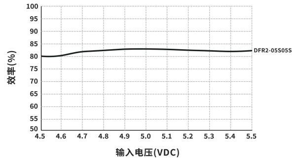
效率 VS 输入电压曲线图 (满载、DFR2-05S05S)
