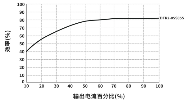
效率 VS 输出负载曲线图 (DFR2-05S05S)
