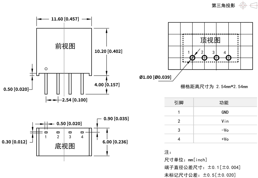
DFR2-xxSxxS 外观尺寸与建议刷版图
