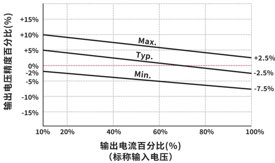
误差包络曲线图 (5/9/12/15/24V 输出)
