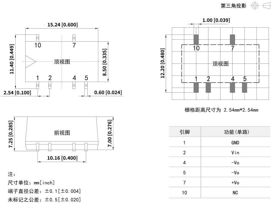
DB1-xxSxxXT 外观尺寸与建议刷版图
