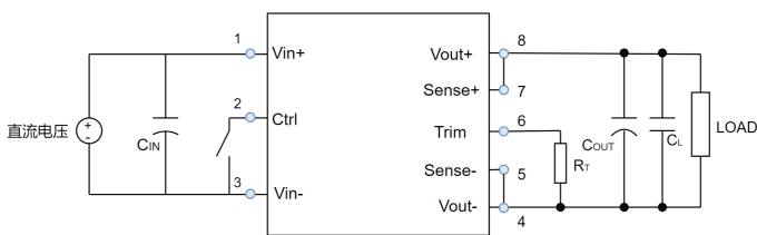
(图 2 输出电压正向调节)
