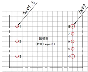
推荐印制板 注：栅格尺寸为2.54*2.54mm
