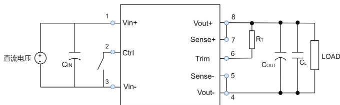
(图 3 输出电压负向调节)
