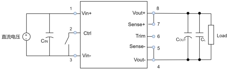
(图 1：典型应用图接线)
