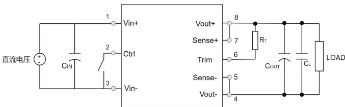
(图 3 输出电压负向调节)
