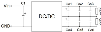
(图 1, 单路输出)
