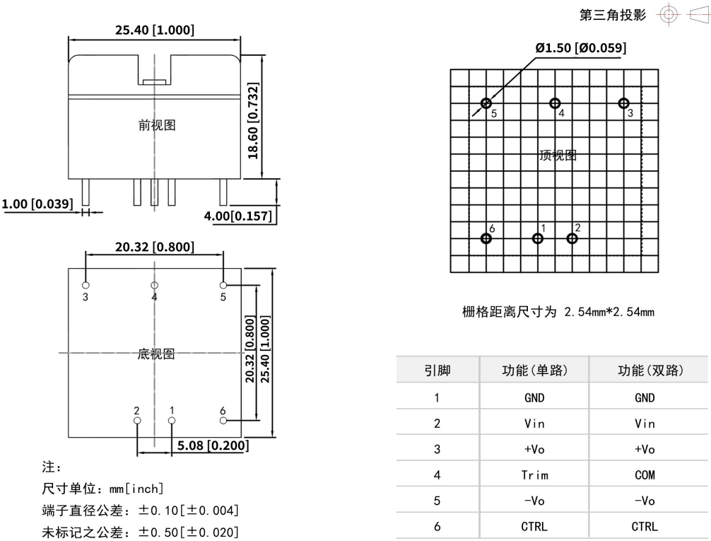
VB20-xxDxxMDH 外观尺寸与建议刷版图
