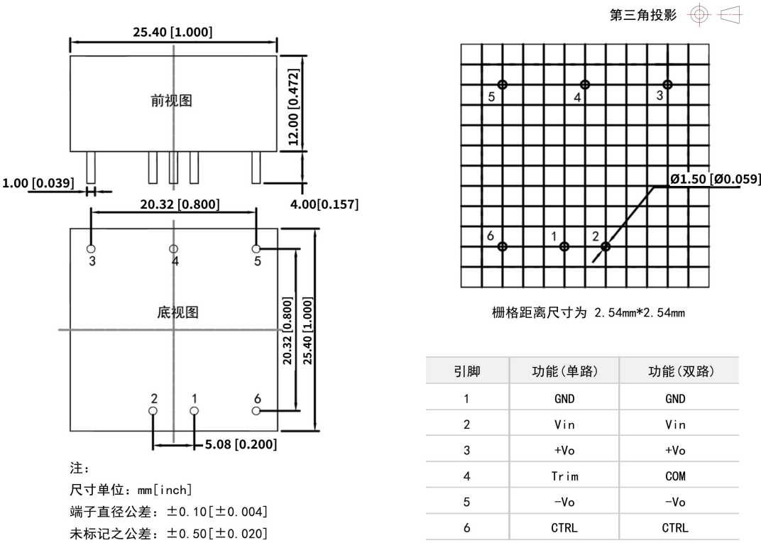
VB20-xxDxxMDH 外观尺寸与建议刷版图
