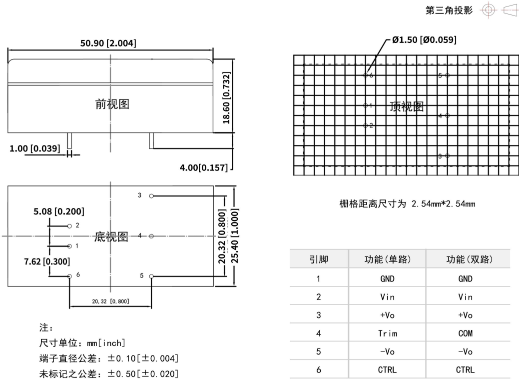
VB20-xxS/DxxLDH 外观尺寸图
