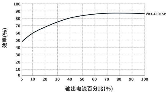
效率 VS 输出负载曲线图 (Vin=48V)
