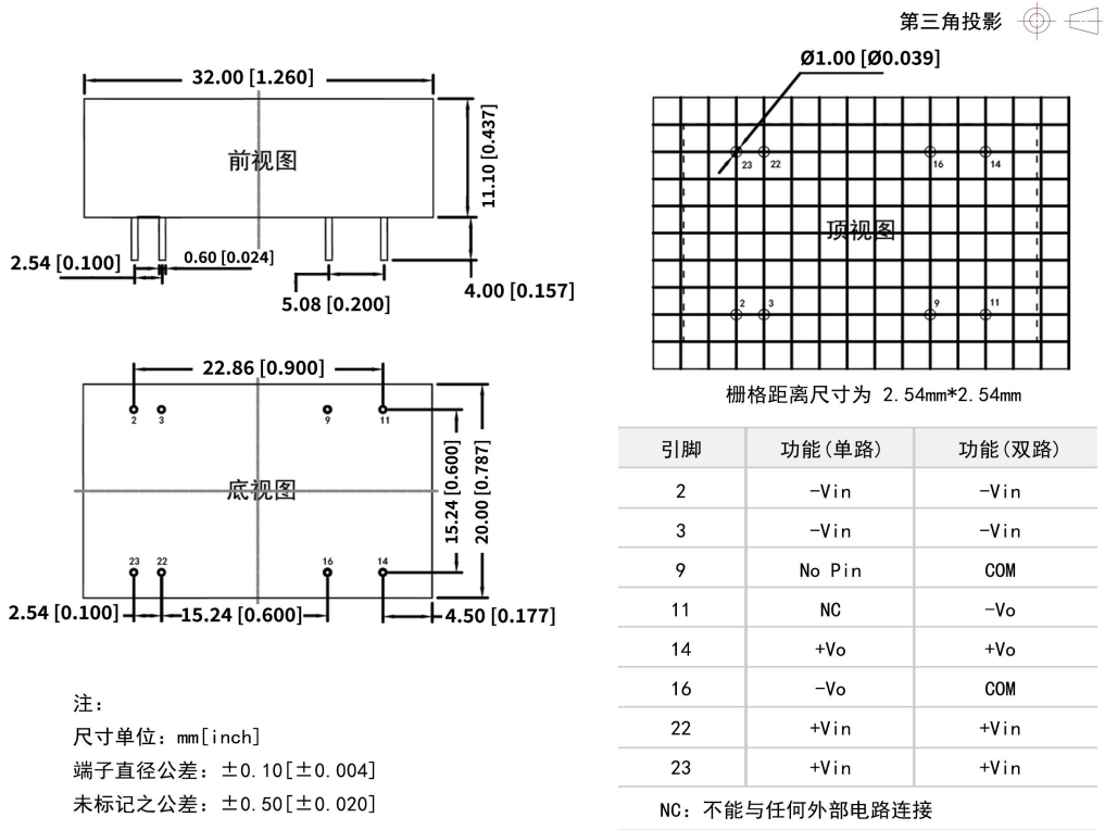
VB3-xxS/DxxP 外观尺寸与建议刷版图
