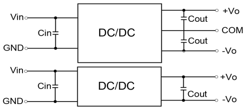
(图 1, 双路/单路输出)
