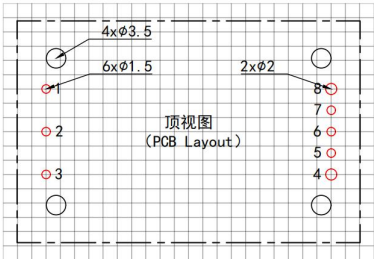
推荐印制板 注：栅格尺寸为2.54*2.54mm
