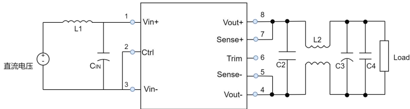
EMI 滤波电路设计与应用
