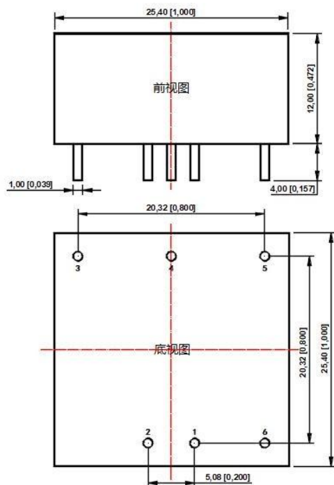
外观尺寸图
