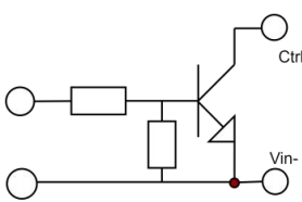
三极管控制方式
