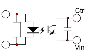
光耦隔离控制方式
