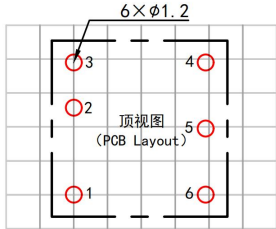
推荐印制板(引脚朝下) 注: 栅格尺寸为2.54*2.54mm
