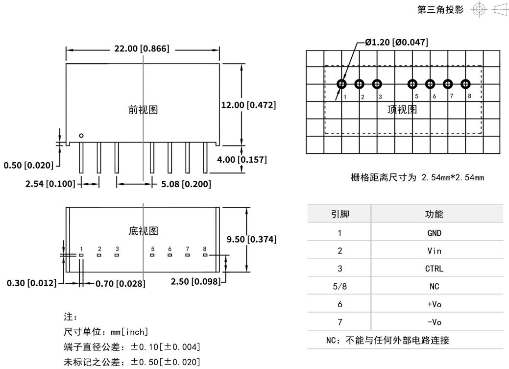
VB6-xxSxxS 外观尺寸与建议刷版图
