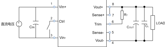
(图3 输出电压负向调节)
