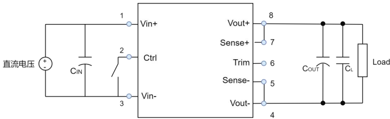
(图 1: 典型应用图接线)
