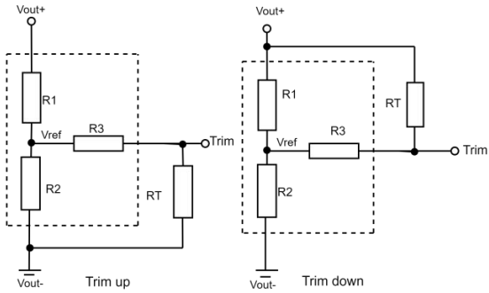
(图4 Trim 的使用电路(虚线框为产品内部))
