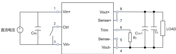
(图2 输出电压正向调节)
